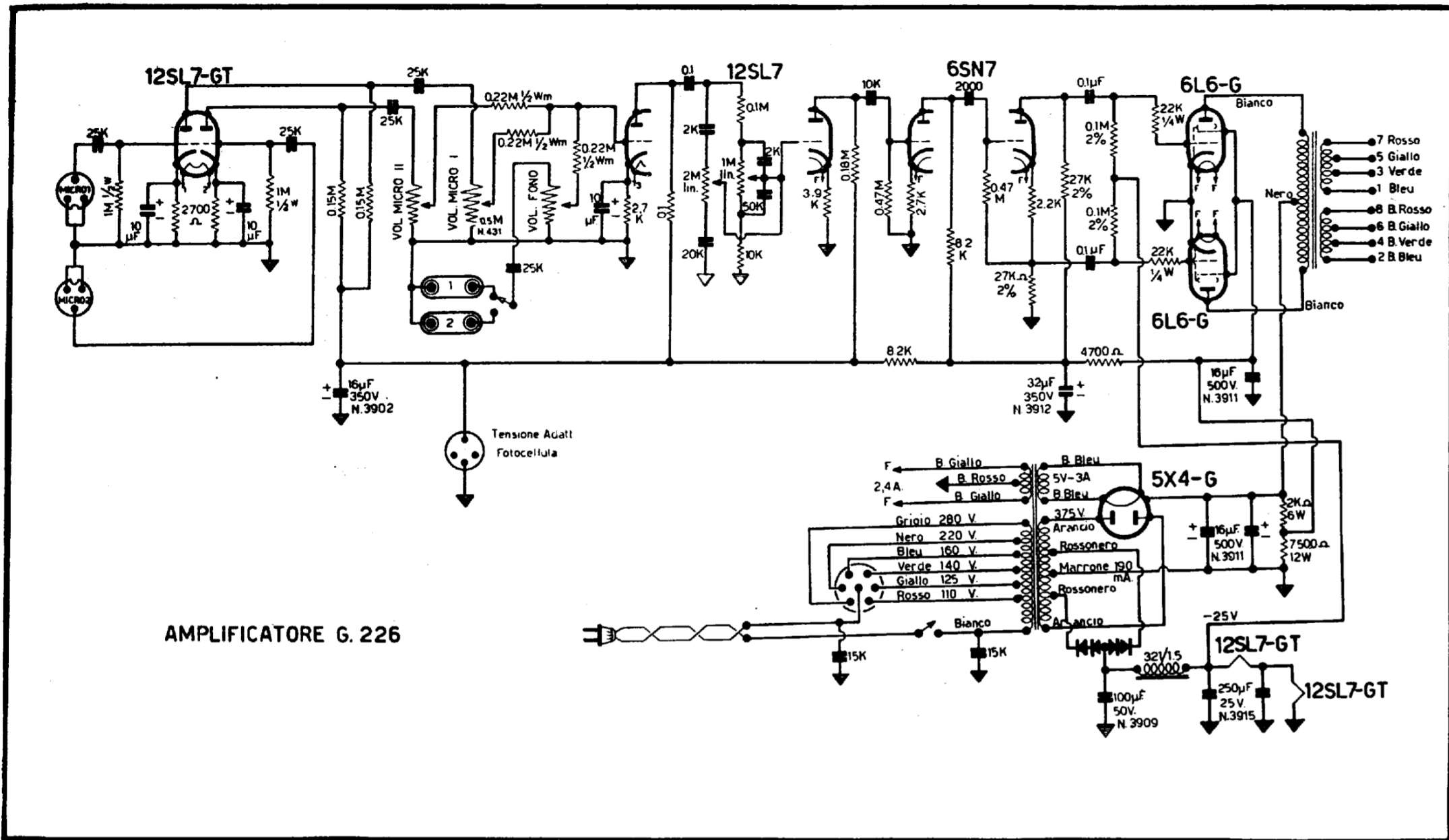
SCHEMA ELETTRICO DELL'AMPLIFICATORE DI POTENZA MOD. G. 226
